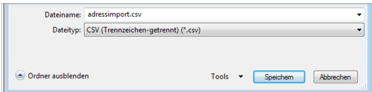
Abbildung 2: Datei Speichern
